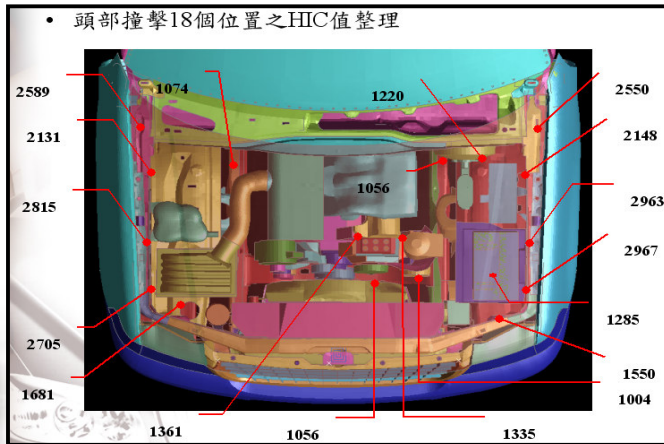
(1)2003/102/EC行人碰撞之頭部CAE分析
