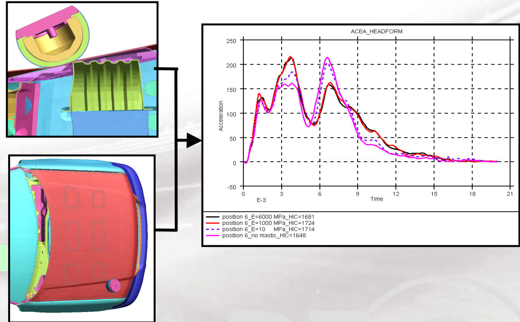
(1)2003/102/EC行人碰撞之頭部CAE分析
