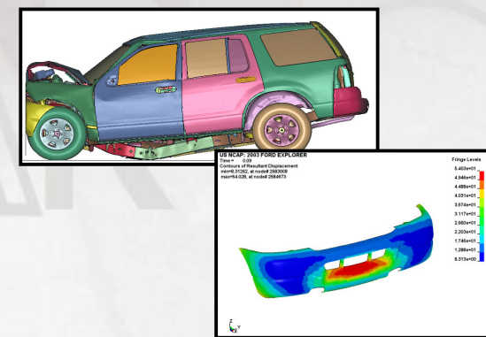
(3)目標車正碰撞及保險桿低速碰撞
