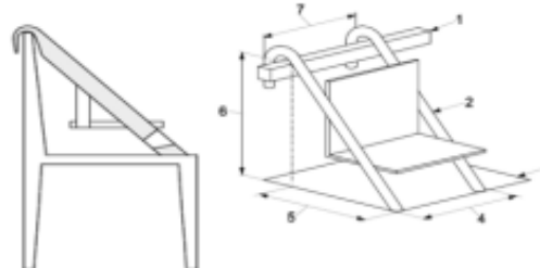
以成人椅背頂部為支撐之椅上架高座
